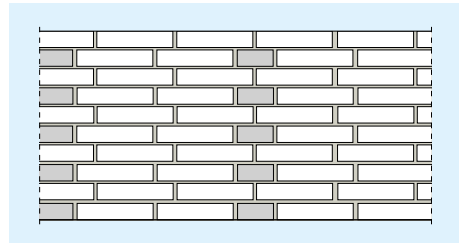
Bild 27 Märkischer Verband – Abwandlung mit Läuferschichten
