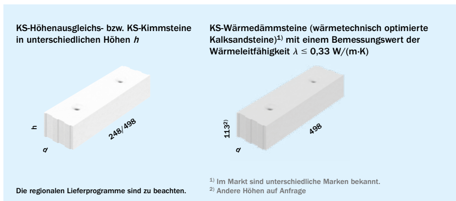
Bild 11 KS-Kimmsteine und KS-Wärmedämmsteine
