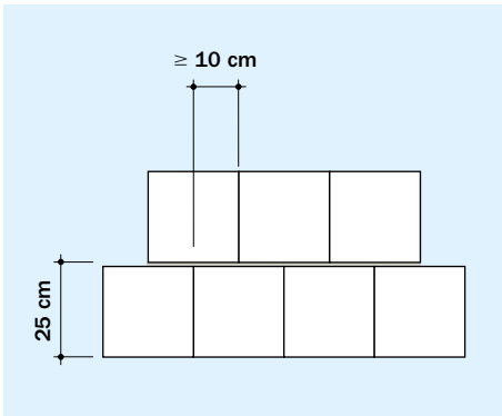
Bild 7 Mindestüberbindemaß I_{oi} für KS-Plansteine
