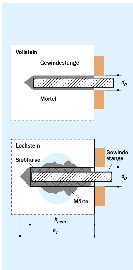
Bild 9 Injektionsdübel in KS-Vollstein und KS-Lochstein
