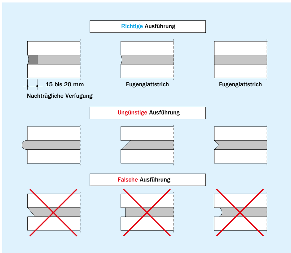
Bild 35 Ausführung von Mörtelfugen in Verblendschalen [3]
