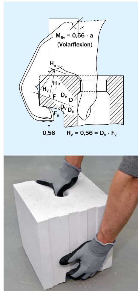
Bild 1 Mittelformatiger Kalksandstein mit optimierter Griffhilfe
