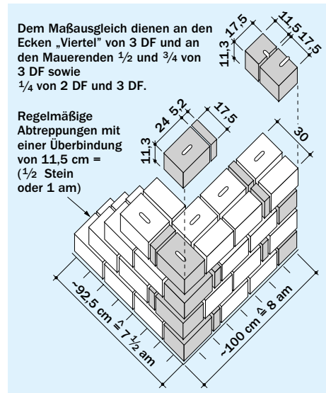
Bild 16 Ecke von 30 cm dicken Wänden aus 2 DF- und 3 DF-Steinen im Verband mit Schnitthugen
