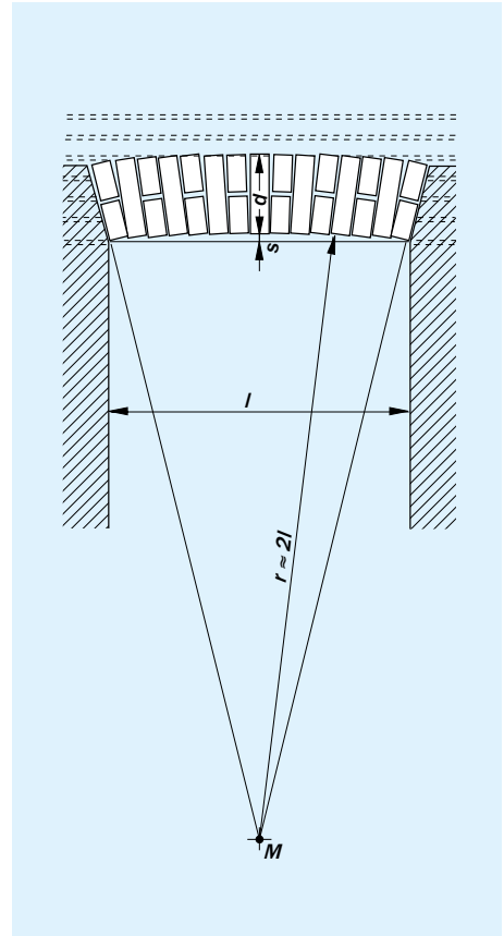
Bild 19 Beim scheitrechten Bogen muss der Bogenstich (Überhöhung) mindestens 2 cm betragen.
