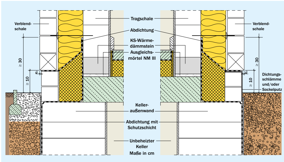
Bild 44 Beispiel für Fußpunktbauweise mit einem Sockel aus Verblendern und Kiesrandstreifen sowie einem verputzten Sockel ohne Kiesrandstreifen
